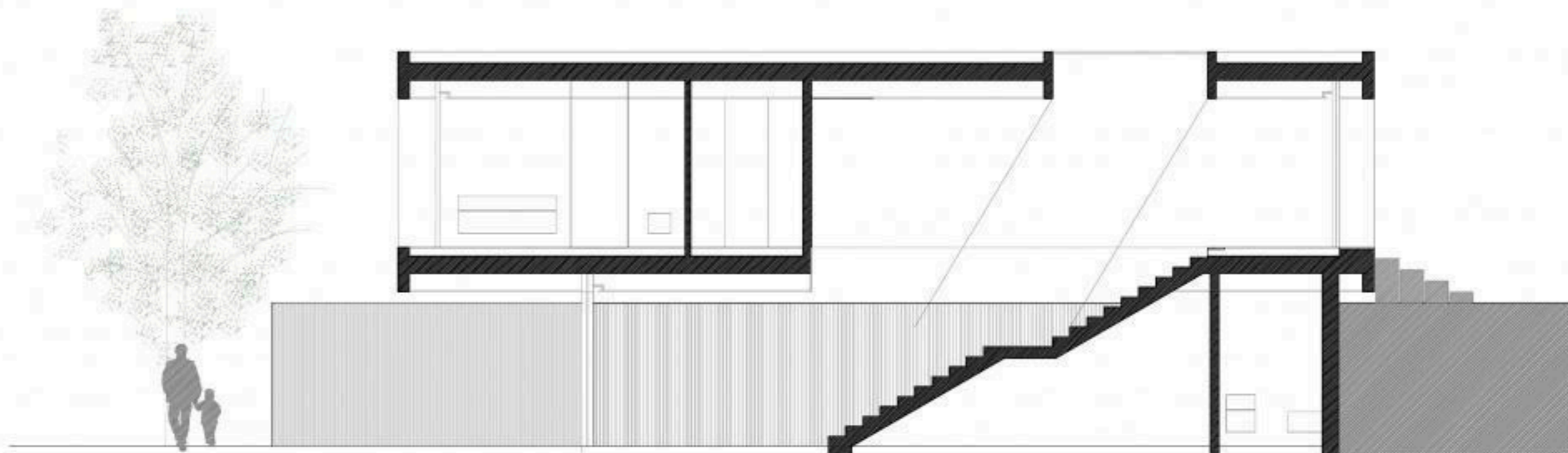
A-A' SECTION SECCIÓN A-A'
